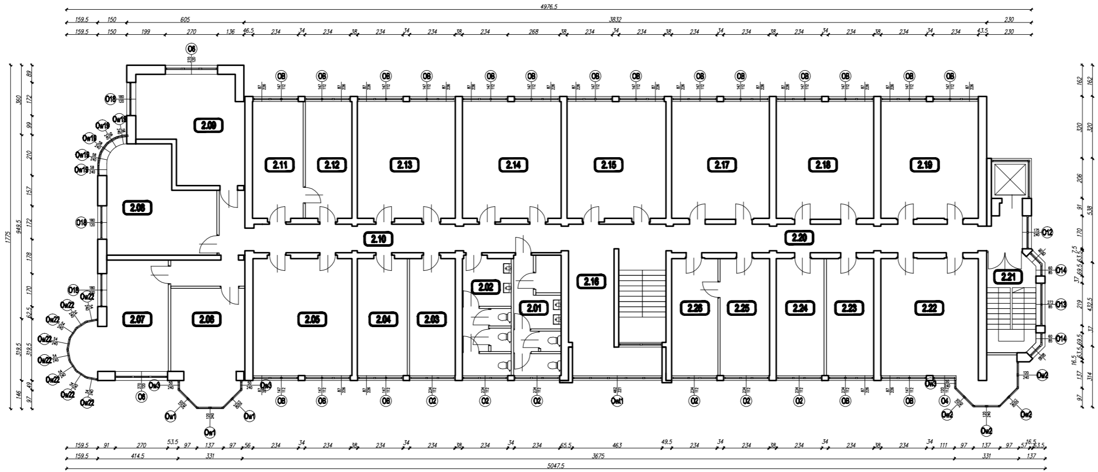
RZUT 2 PIĘTRA
