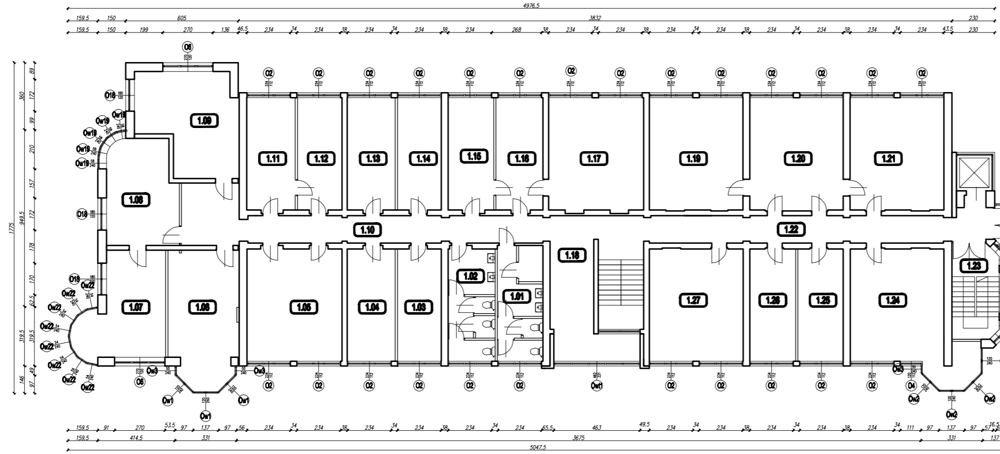
RZUT 1 PIĘTRA
