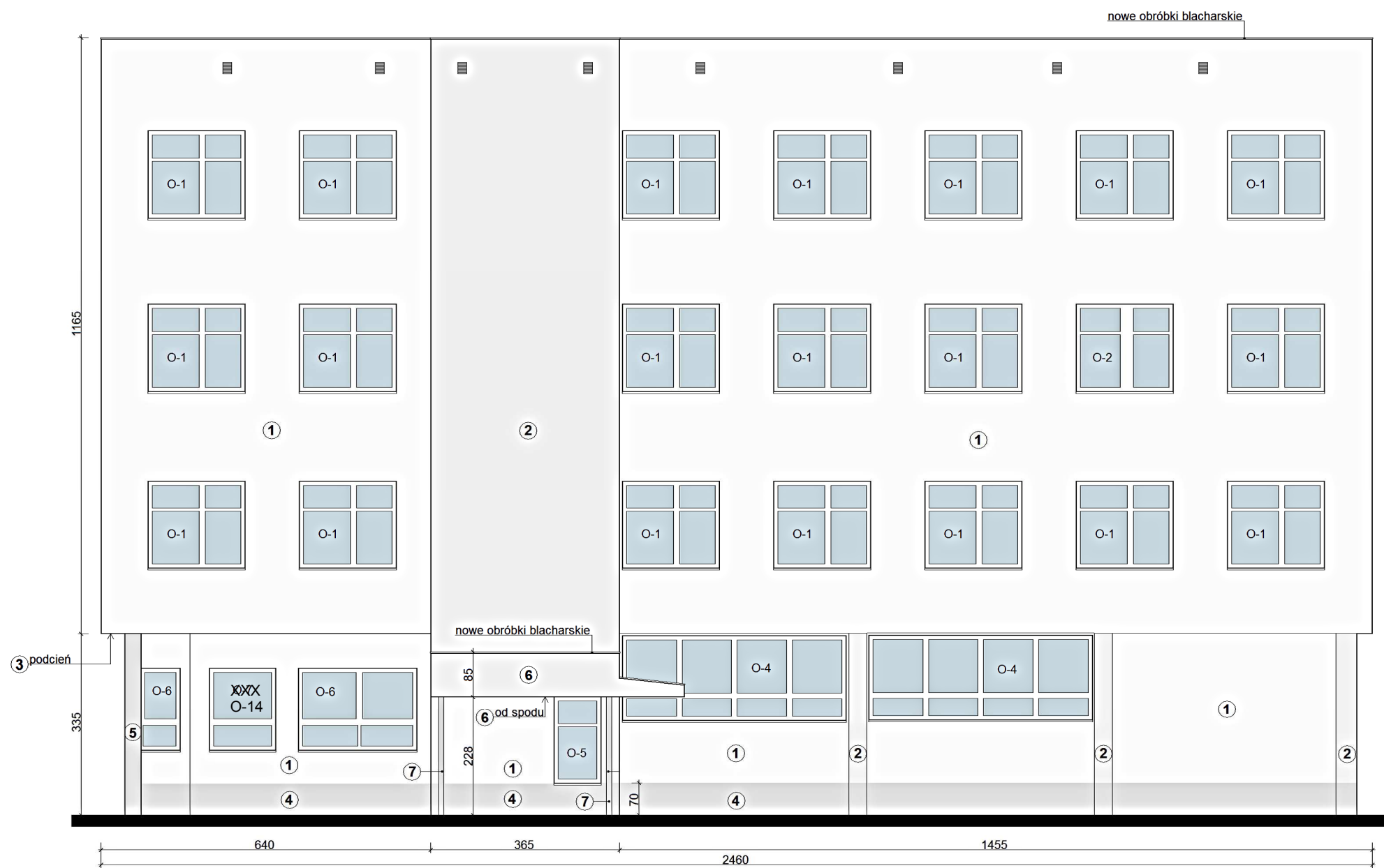
ELEWACJA POŁUDNIOWA
